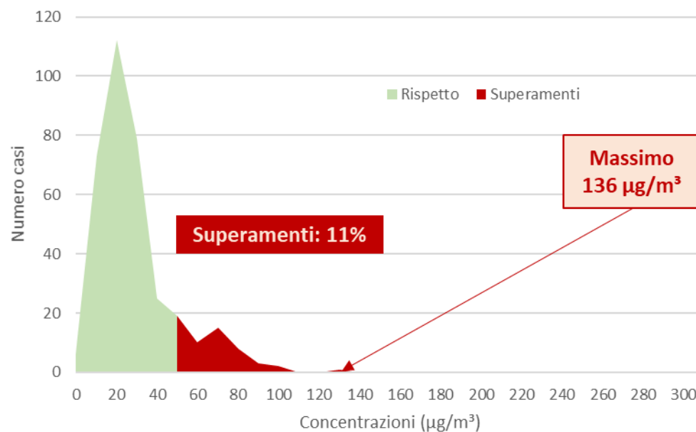
PM10 Milano-Verziere 2016
