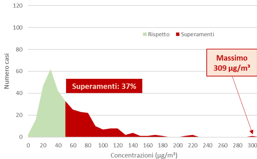
PM10 Milano-Verziere 2016
