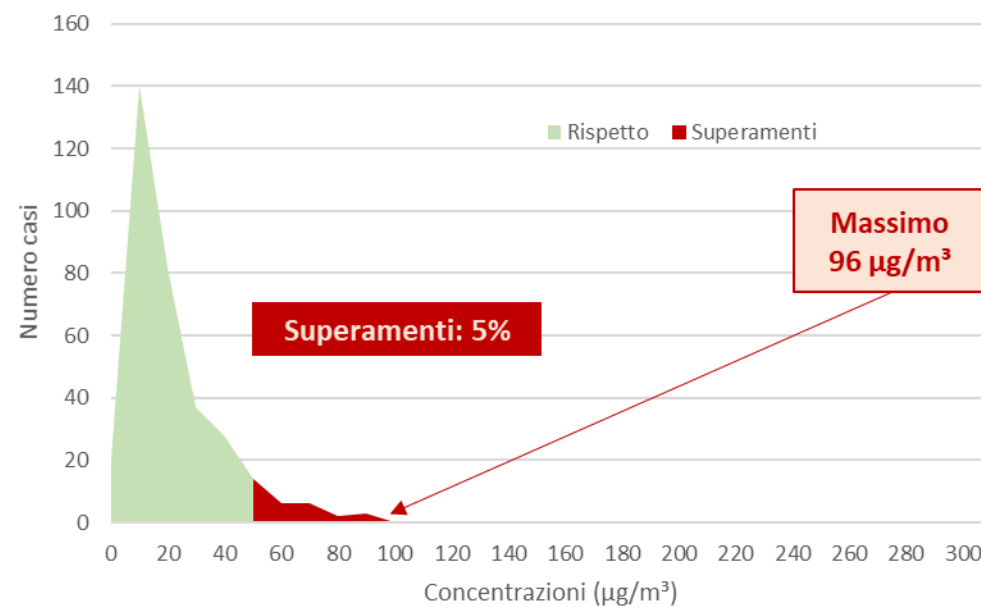
PM10 Milano-Verziere 2021
