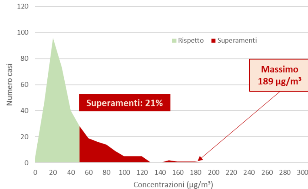
PM10 Milano-Verziere 2021
